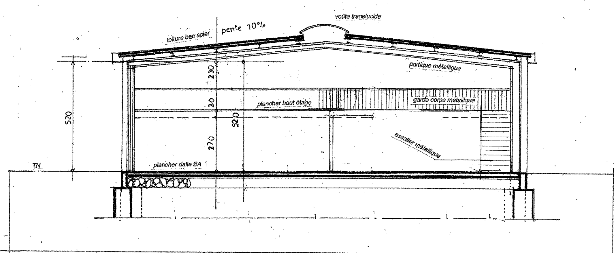
COUPE AA 1/100
